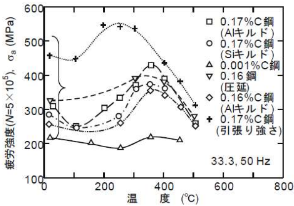
疲労強度の温度依存性
