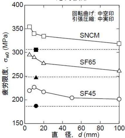
疲労限度の寸法効果
