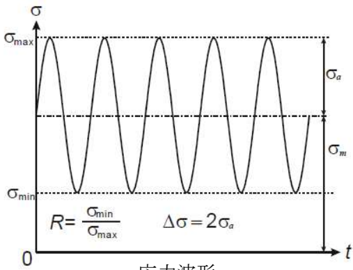
応力波形
