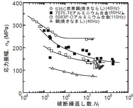
S-N 曲線
