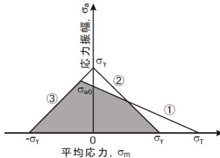
疲労限度に及ぼす平均応力の影響
