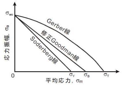
疲労限度に及ぼす平均応力の影響
