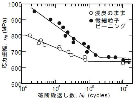
疲労強度に及ぼす浸炭処理の影響
